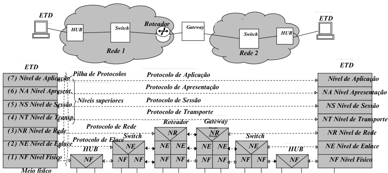
Figura 9 - Conexão entre dois ETDs passando por duas redes e diferentes equipamentos intermediários. (a) Topologia e (b) modelagem da topologia segundo o MR-OSI
