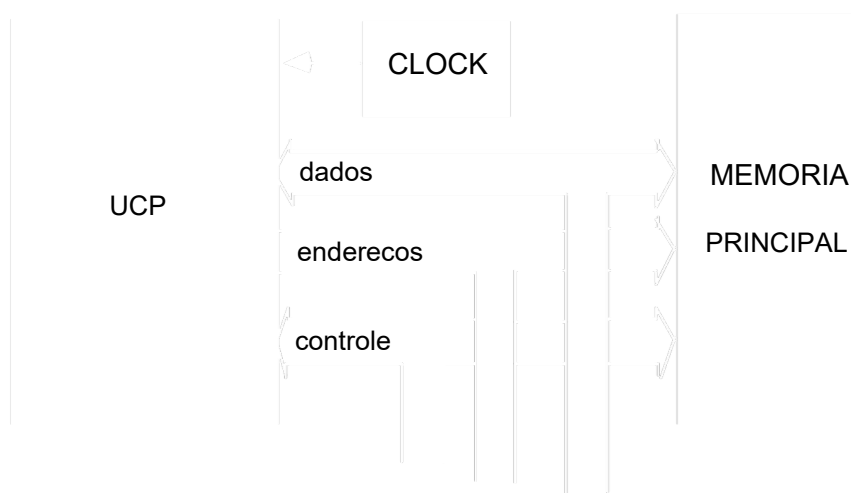
Figura 2 - Barramento
